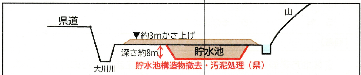
A-A' 断面
