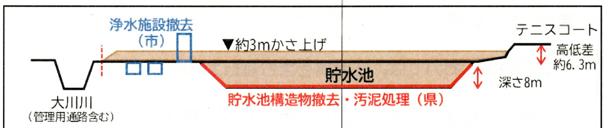
B-B' 断面
